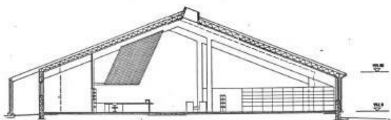
LEIKKAUS D-D
