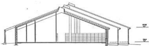
LEIKKAUS C-C
